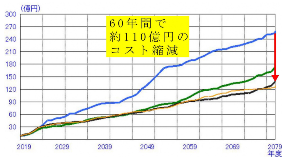
図-1 シナリオごとの修繕費の推移
