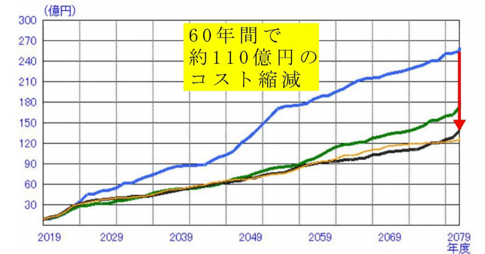
凡例 トータルコスト最小 ①予防保全型 ②事後保全型 ③大規模補修・更新型
