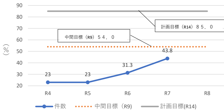
3-2-1 橋梁補修着手率（補修着手数/補修必要数）
